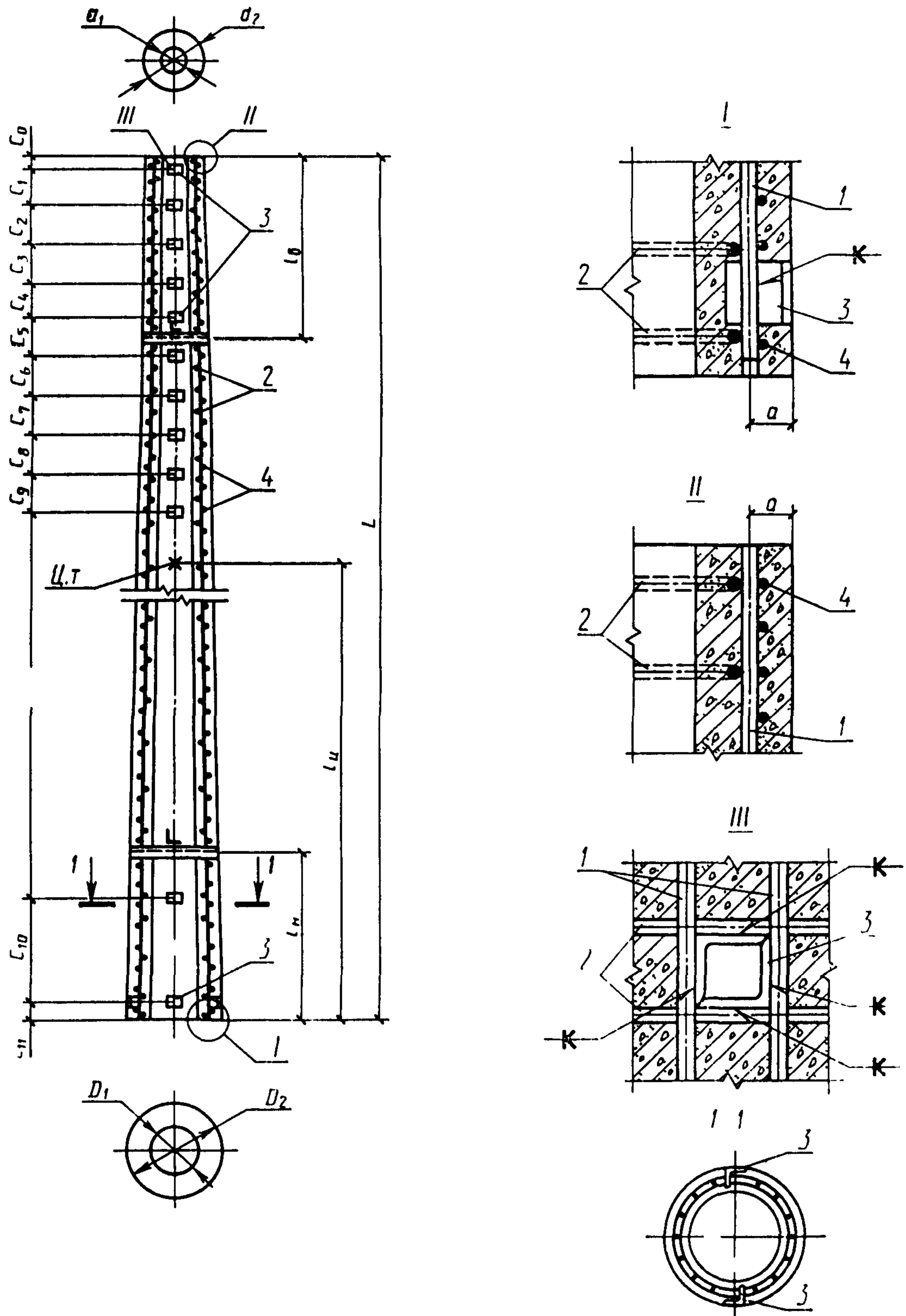
1—продольная арматура, 2—монтажные кольца, 3—закладные изделия, 4—спираль; a —расстояние от наружной поверхности стойки до оси продольной арматуры, C_0 — C_{11} —вязка закладных изделий, ц т — центр тяжести; L —длина стойки, l_{ц} —расстояние до центра тяжести, l_{н} , l_{в} —расстояния от мест установки диафрагм, D_1 , d_1 —внутренние диаметры стойки, D_2 , d_2 —наружные диаметры стойки
