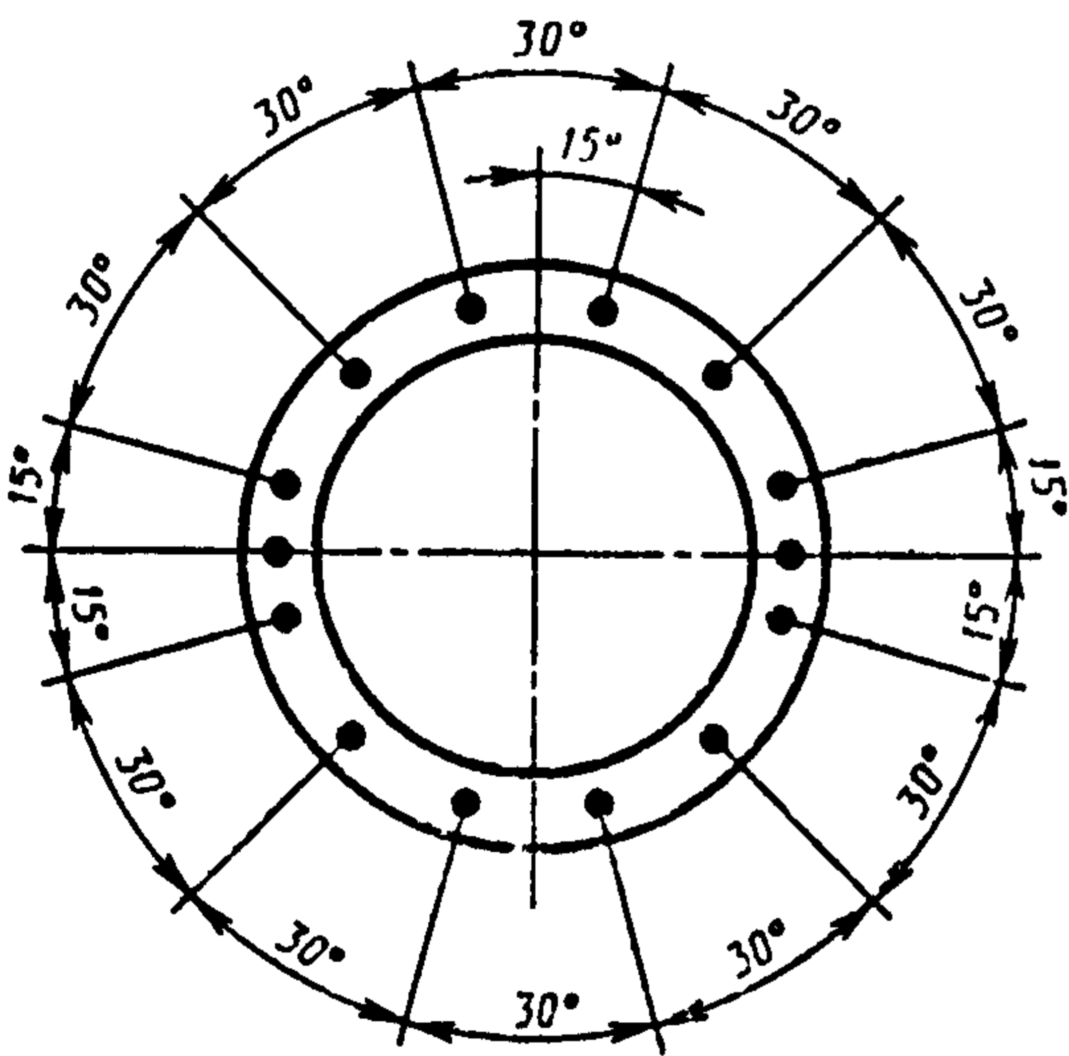
СК22.3—1.0, СК22.3—1.1, СК22.3—1.2
